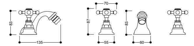
7392 Batteria bidet 3 fori con bocca s. a. Three holes bidet mixer with pop up waste
