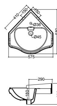
1032 Lavabo angolo monoforo One hole corner basin
