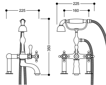
7396 Coppia colonnine cm 10 per attacco bordo vasca Pair of columns cm 10 for deck mounting
