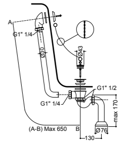
1053 Colonna di scarico esterna per vasca Visible bath-tub waste-pipe
