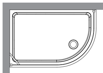
9137 Cabina doccia semicircolare DX per piatto doccia 80x120 DX. Apertura utile 63 cm, altezza 180 cm. Right semicircular shower enclosure for right shower-tray 80x120. Usable opening 63 cm, height 180 cm.
