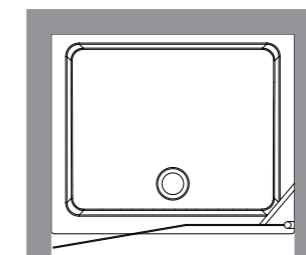
9140 Porta battente SX con fisso in linea per piatto doccia 80x92 nicchia. Apertura utile 54 cm, altezza 180 cm. Left shower door for niche installation shower-tray 80x92. Usable opening 54 cm, height 180 cm.
