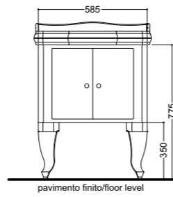
7361 Mobile chiuso laccato nero lucido per lavabo 69 Bright-black cabinet for washbasin 69 lacquer finish
