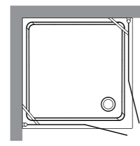
9145 Cabina doccia DX/SX a due porte battenti e fisso in linea per piatto doccia 90x90 quadro. Apertura utile 36 cm più anta, altezza 180 cm. Reversible shower enclosure with two door for corner shower-tray 90x90. Usable opening 36 cm each door, height 180 cm.
