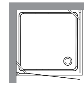
9146 Cabina doccia DX con porta battente e fisso laterale per piatto doccia angolare 90x90 quadro. Apertura utile 72 cm, altezza 180 cm. Right shower enclosure with door for corner shower-tray 90x90. Usable opening 72 cm, height 180 cm.
