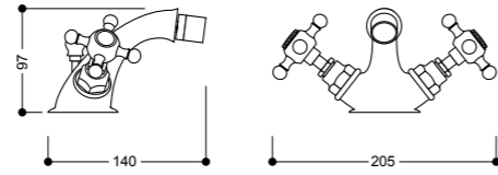
7390 Batteria bidet monoforo s. a. One hole bidet mixer with pop up waste
