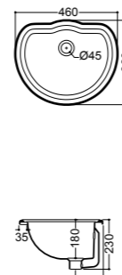
1031 Lavabo incasso 46x38 Inset basin 46x38
