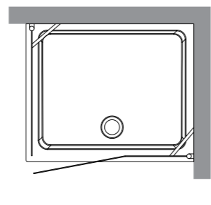
9142 Cabina doccia SX con porta battente in linea e fisso laterale per piatto doccia 80x96 SX apertura lato 96. Apertura utile 54 cm, altezza 180 cm. Left shower enclosure with door for left shower-tray 80x96 opening on 96 side. Usable opening 54 cm, height 180 cm.
