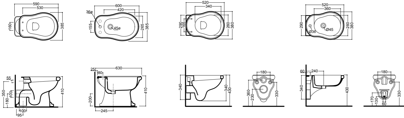
1010 Vaso scarico suolo "S" Wc pan floor outlet
