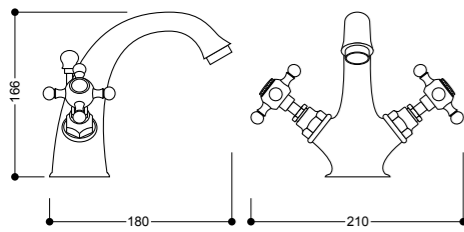
7389 Batteria lavabo monoforo s. a. One hole basin mixer with pop up waste
