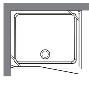
9141 Cabina doccia DX con porta battente in linea e fisso laterale per piatto doccia 80x96 DX apertura lato 96. Apertura utile 54 cm, altezza 180 cm. Right shower enclosure with door for right shower-tray 80x96 opening on 96 side Usable opening 54 cm, height 180 cm.
