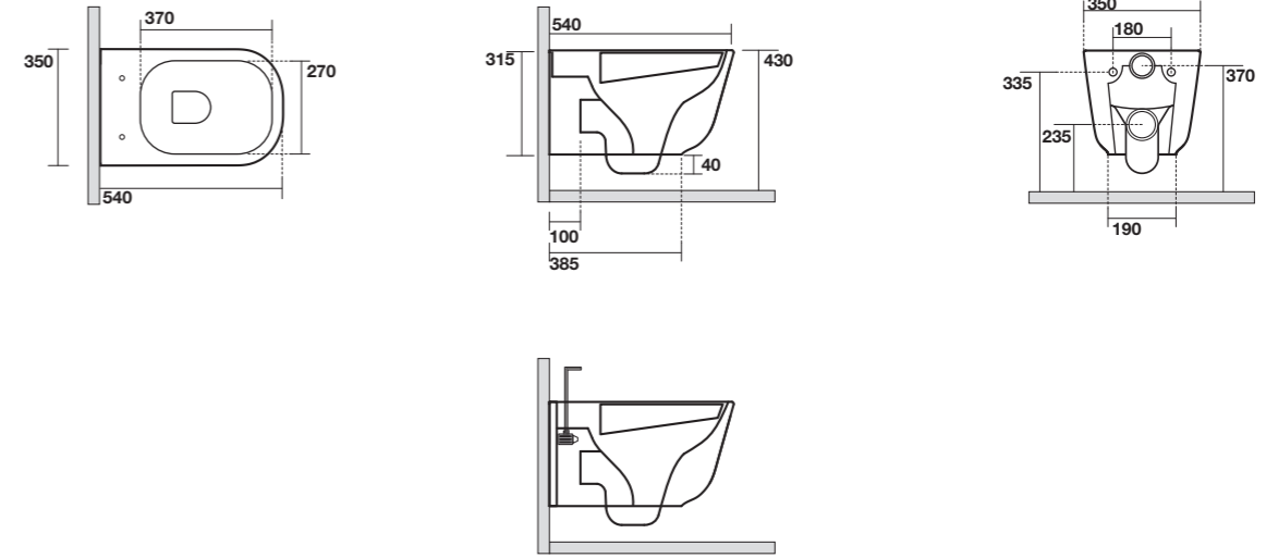
5115 Vaso sospeso completo di protezione acustica e antiurto e fissaggio WB9N Wall hung wc, sound and shock proof plate and fixing screws WB9N included
